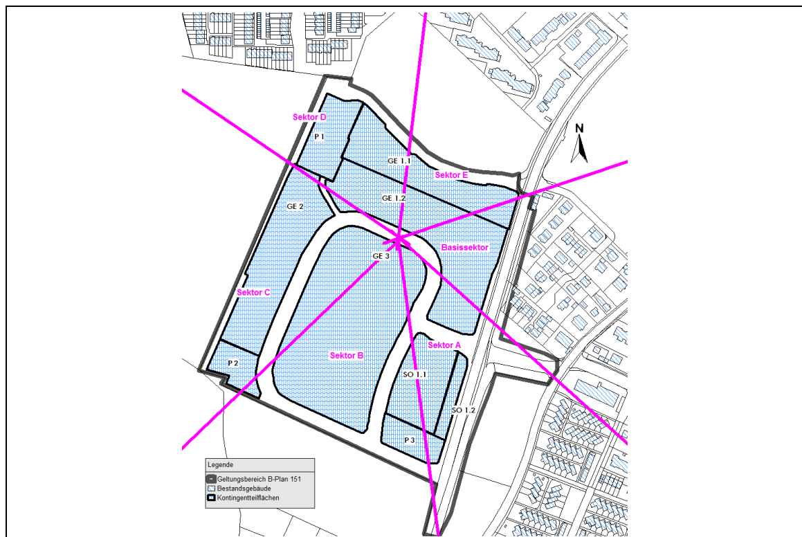
Abbildung 5: Anlagenlärm – Emissionskontingentierung, Zusatzkontingente
